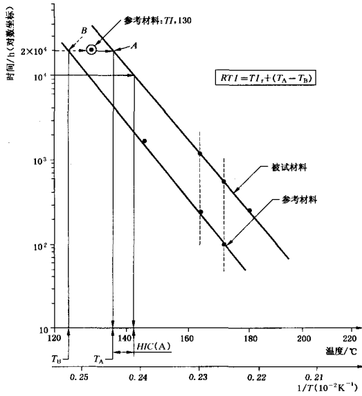
图3 耐热图—相对温度指数-半差
