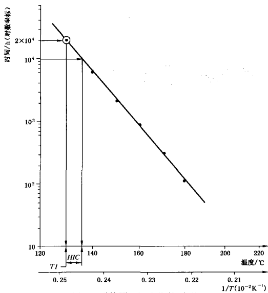
图2 耐热图—温度指数-半差
